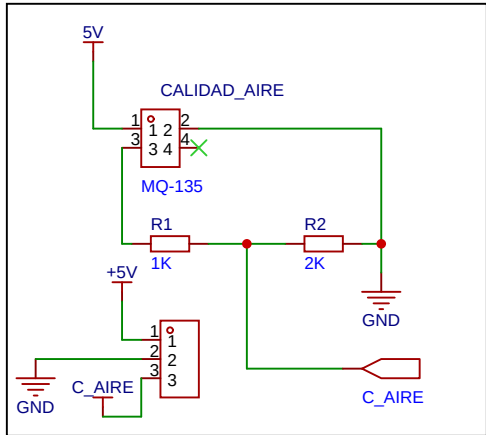
SENSOR DE CALIDAD DEL AIRE MQ-135
