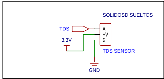
SENSOR DE SÓLIDOS DISUELTOS TDS
