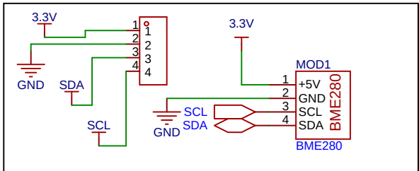
SENSOR DE PRESIÓN, TEMPERATURA Y HUMEDAD BME280
